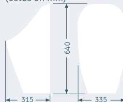
Dimensions « ceramicC2 » (cotes en mm)
