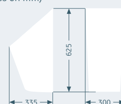
Dimensions « inox » (cotes en mm)
